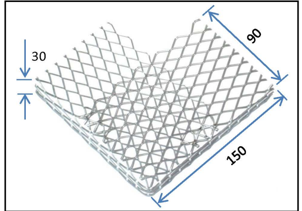
C - LATH ( 30 x 90 x 150 ) 30 x 90 x 225 주문생산규격
